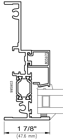
Fixed Jamb
