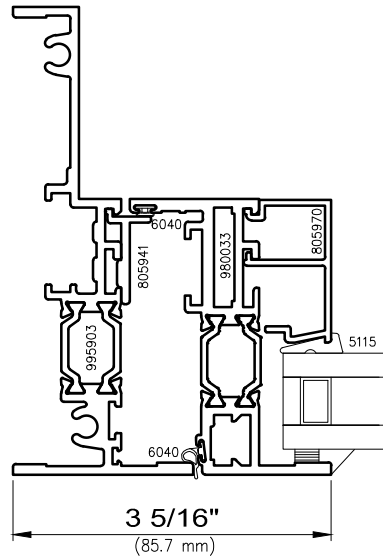
PI Jamb
