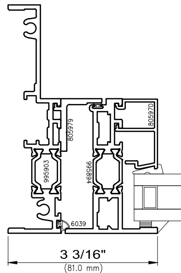
PO Jamb
