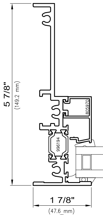
8 Fixed Jamb Inside Slide
