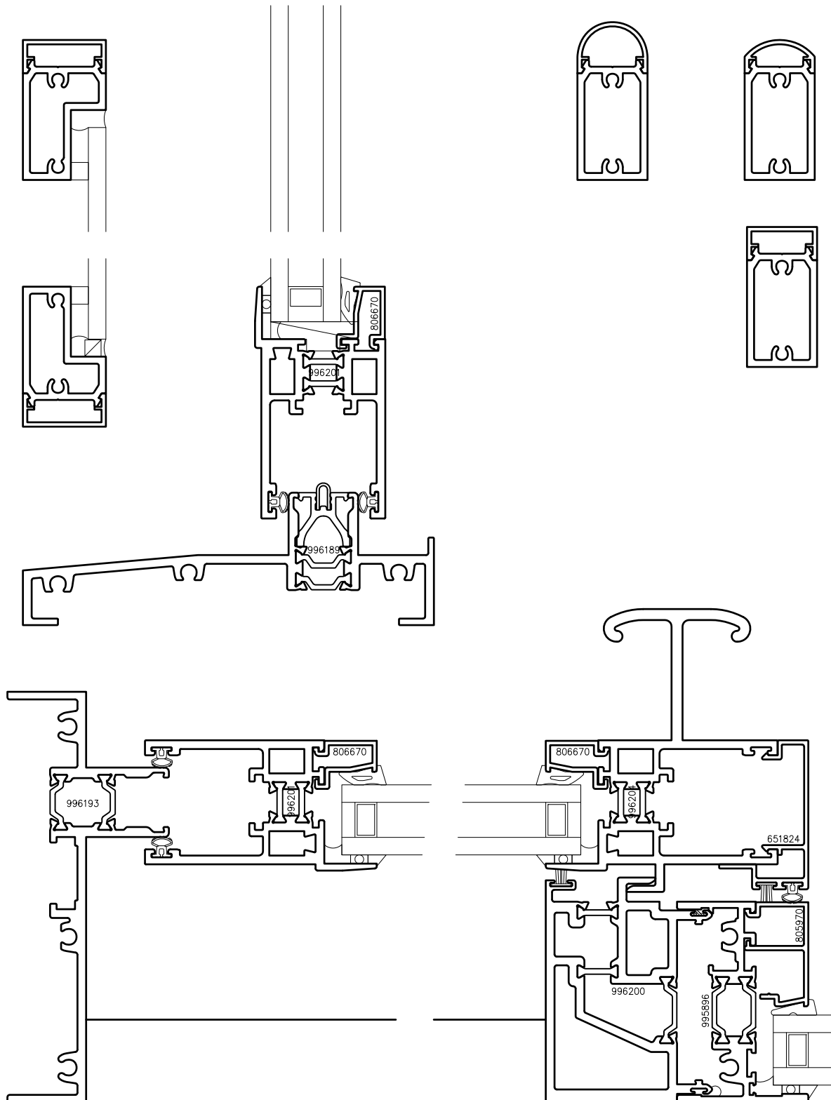
Juliet Balcony
